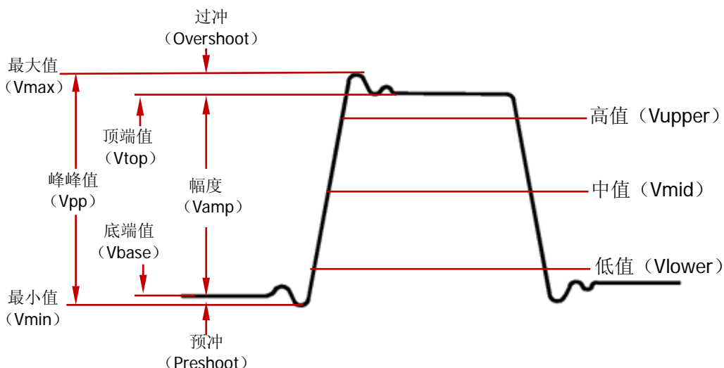
图 6-5 电压参数
