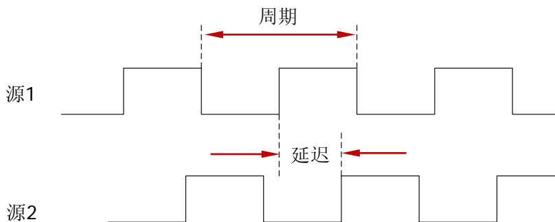
图 6-4 延迟和相位
