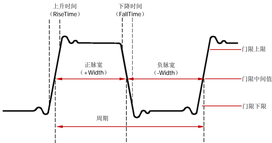
图 6-3 时间参数
